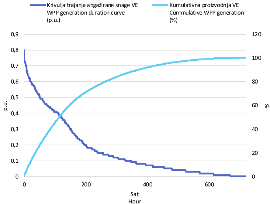
Slika 3 Krivulja trajanja angažirane snage svih VE i kumulativna proizvodnja VE u rujnu 2025. godine u jediničnim vrijednostima
