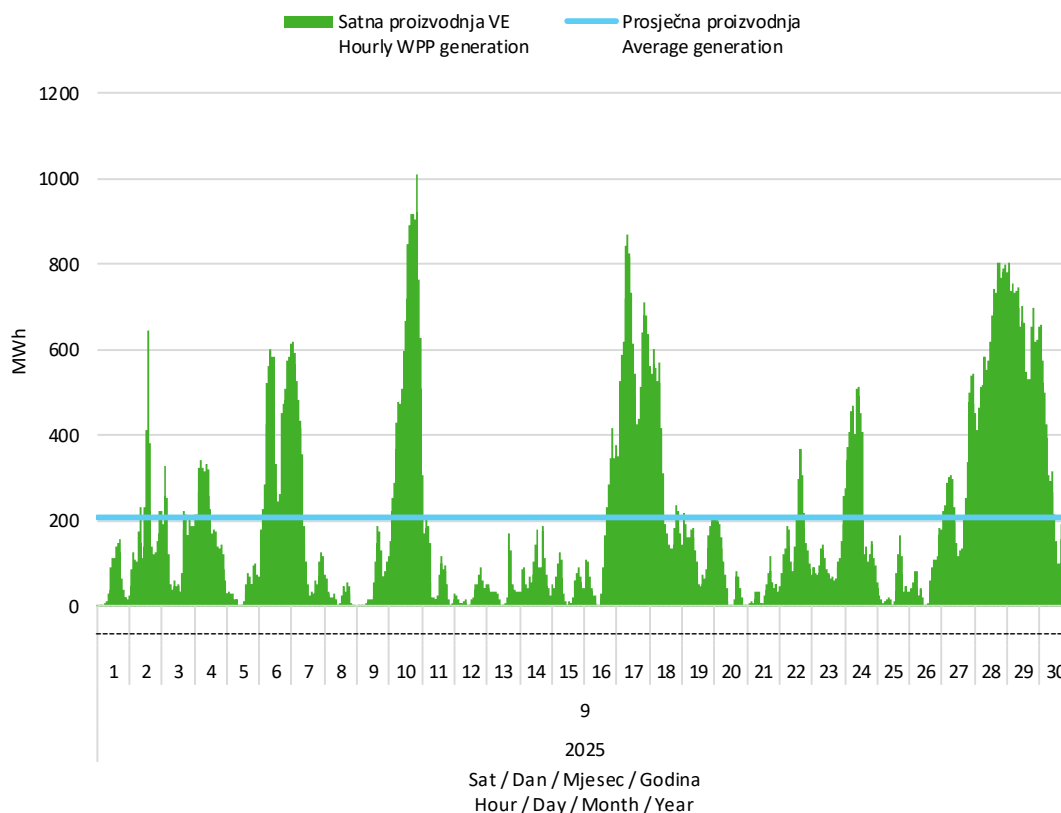
Slika 2 Satna proizvodnja svih vjetroelektrana u rujnu 2025. godine
