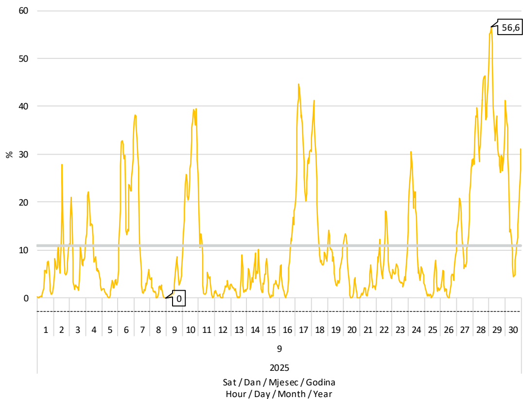
Slika 8 Udio proizvodnje vjetroelektrana u pokrivanju satnog opterećenja elektroenergetskog sustava u rujnu 2025. godine
