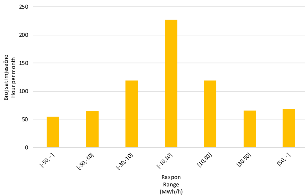
Slika 10 Statistička raspodjela satnih promjena proizvodnje VE u rujnu 2025. godine
