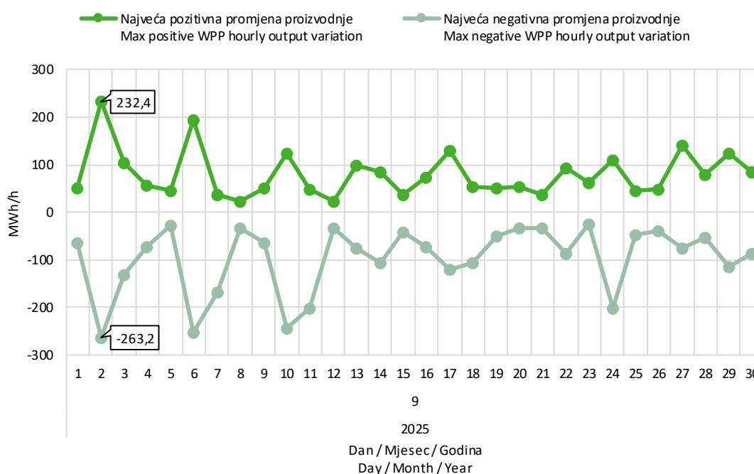
Slika 9 Maksimalna pozitivna i maksimalna negativna promjena satne proizvodnje VE u rujnu 2025. godine
