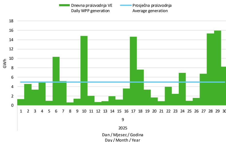
Slika 5 Dnevna proizvodnja svih vjetroelektrana u rujnu 2025. godine
