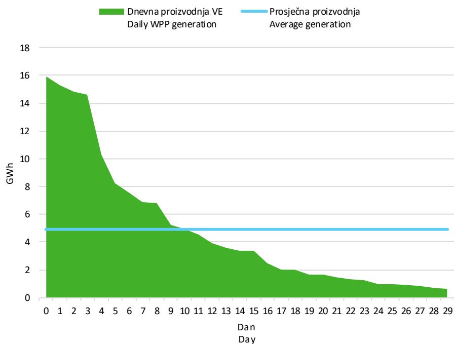
Slika 6 Krivulja trajanja dnevne proizvodnje vjetroelektrana u rujnu 2025. godine
