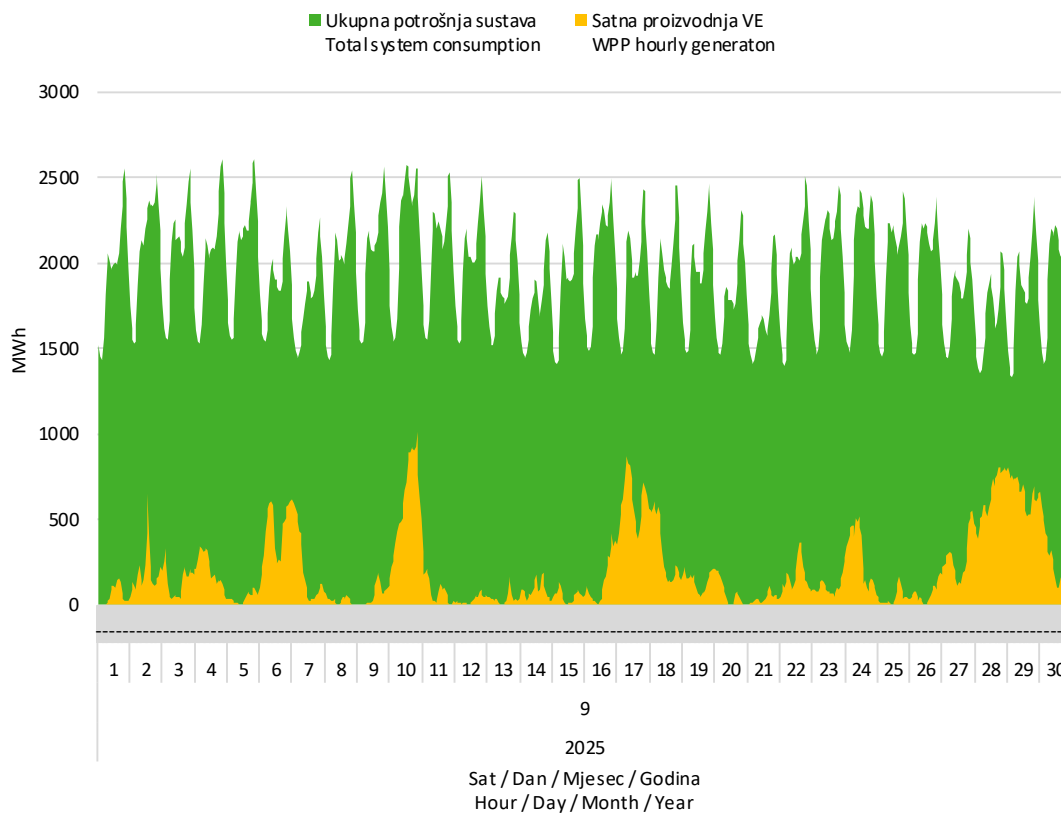
Slika 7 Usporedba satnog dijagrama opterećenja sustava i proizvodnje vjetroelektrana u rujnu 2025. godine
